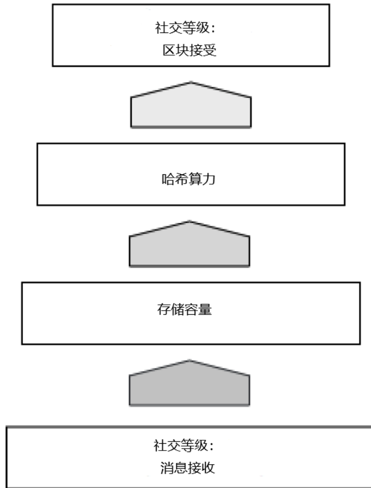
图5：挖矿的条件
